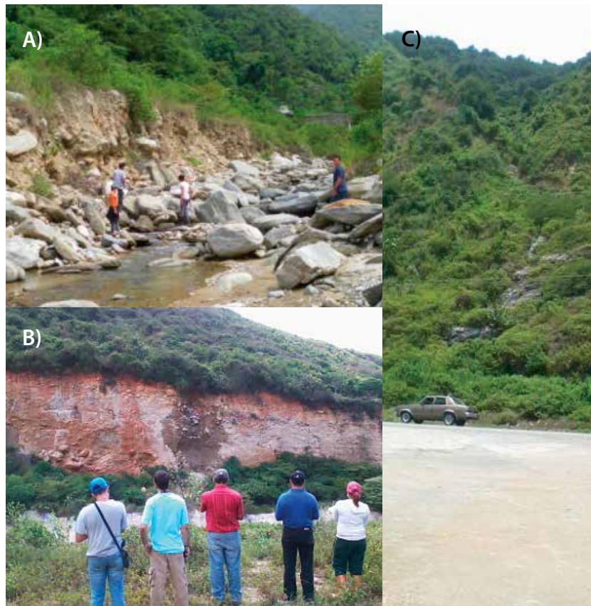
Figura 4. Algunos rasgos geomorfológicos: A) depósitos de abanico aluvial disectados (abanico de la quebrada Camurí Chiquito), B) aluviones colgados (valle de la quebrada San Julián), y C) valles colgados (Carmen de Uria), que evidencian el control tectónico sobre el relieve.
