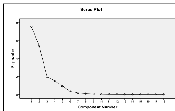
Figura 9. Gráfico de sedimentación de los componentes principales de los parámetros morfométricos del relieve.
