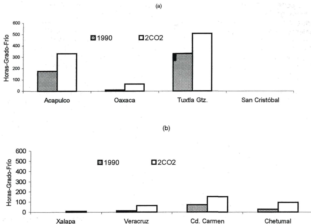
Figura 5. Necesidades anuales de enfriamiento a) en ciudades del transecto sur, y b) en ciudades del transecto norte.
