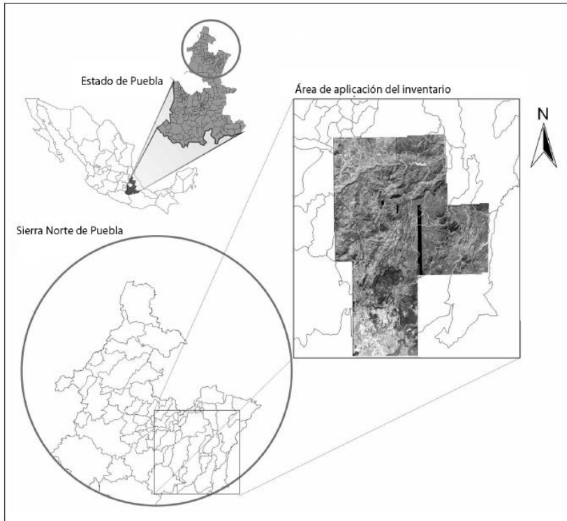
Figura 3. Delimitación del área de aplicación del inventario de procesos de remoción en masa, Sierra Norte de Puebla.
