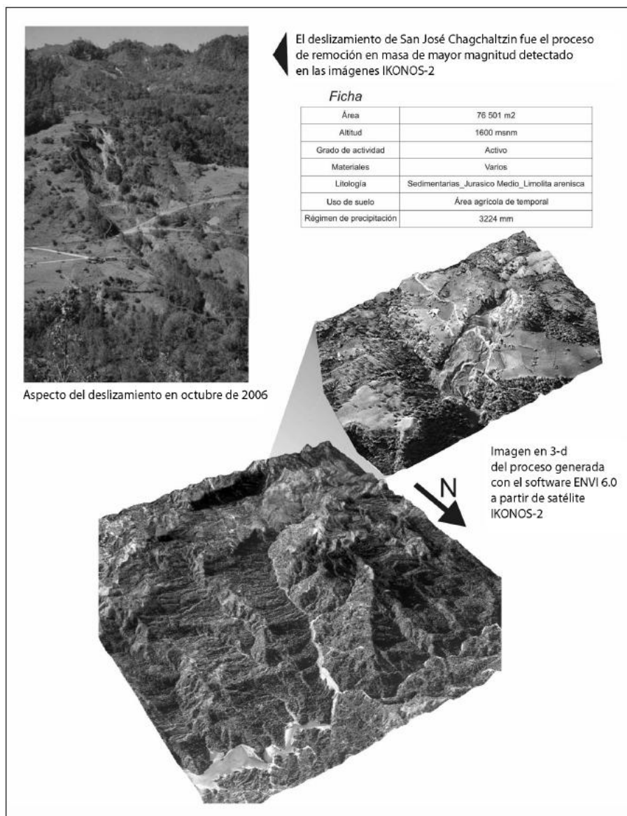
Figura 5. Identificación e información del deslizamiento de San José Chagchaltzin, municipio de Tlatlauquitepec.
