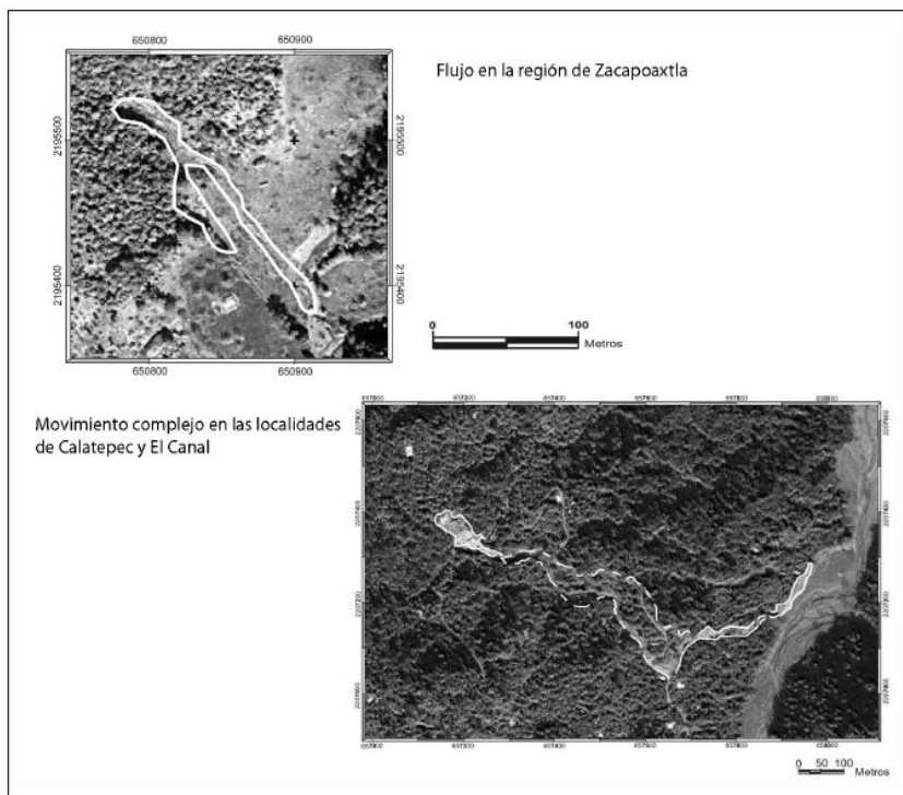
Figura 4. Identificación de procesos de remoción en masa mediante el análisis de imágenes de satélite IKONOS-2.
